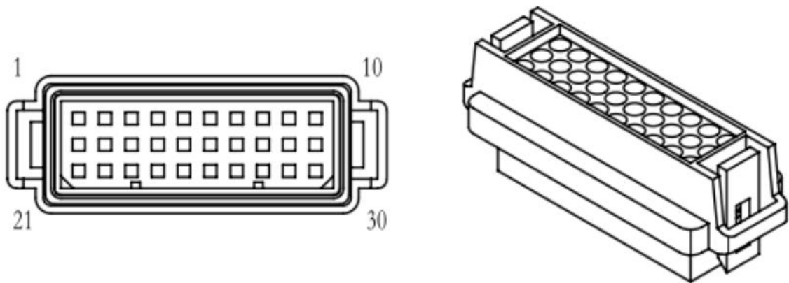
控制器接口定义（30Pin ZT2023 1.1*1.1*19.3）（母端 ZT2024-A）
